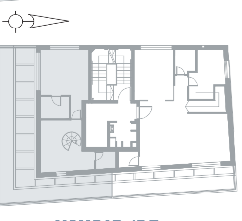
קומת גג
